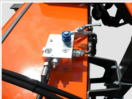
Bloc hydraulique et vanne d'arrêt
